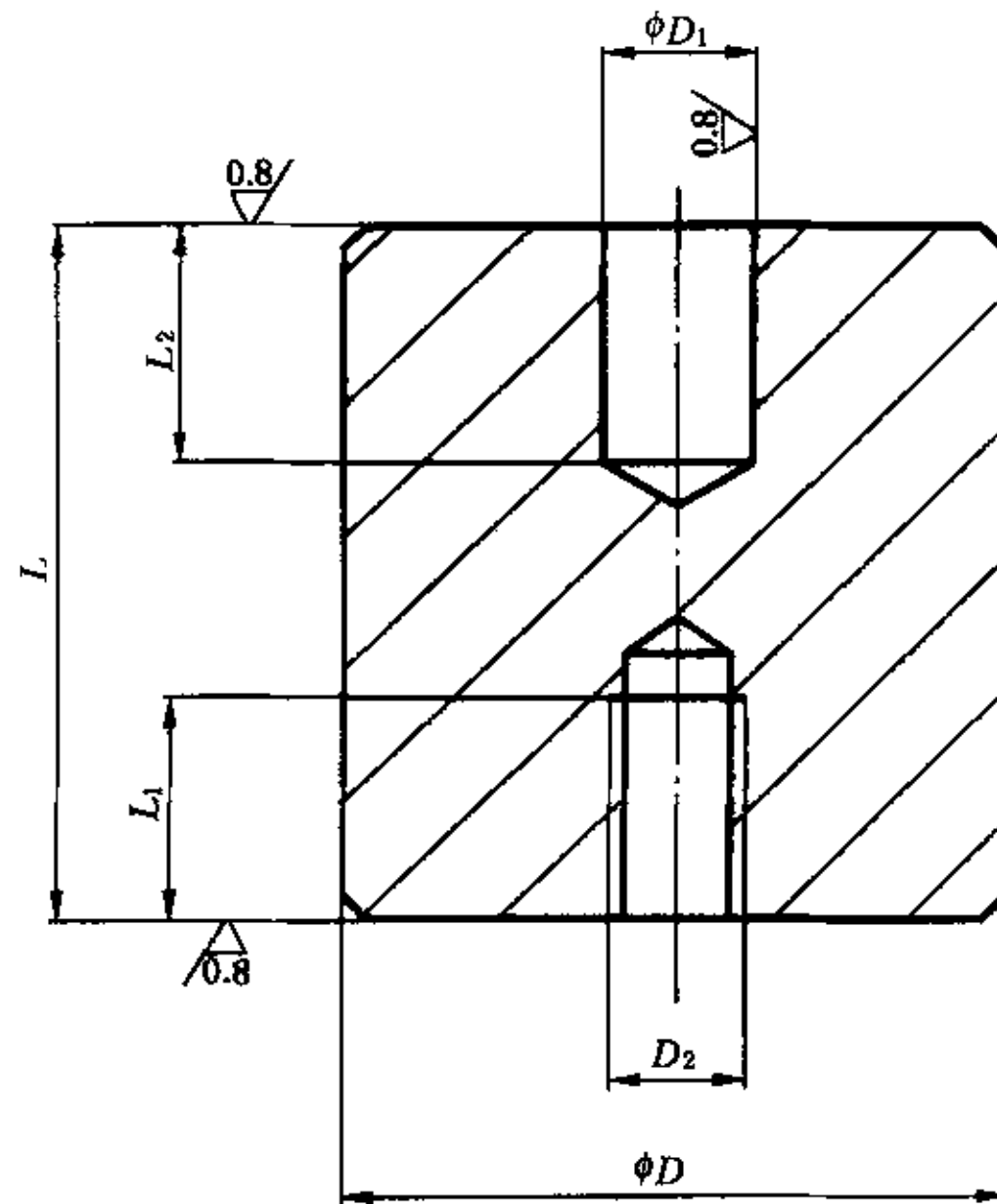
图 2 B型支承柱
